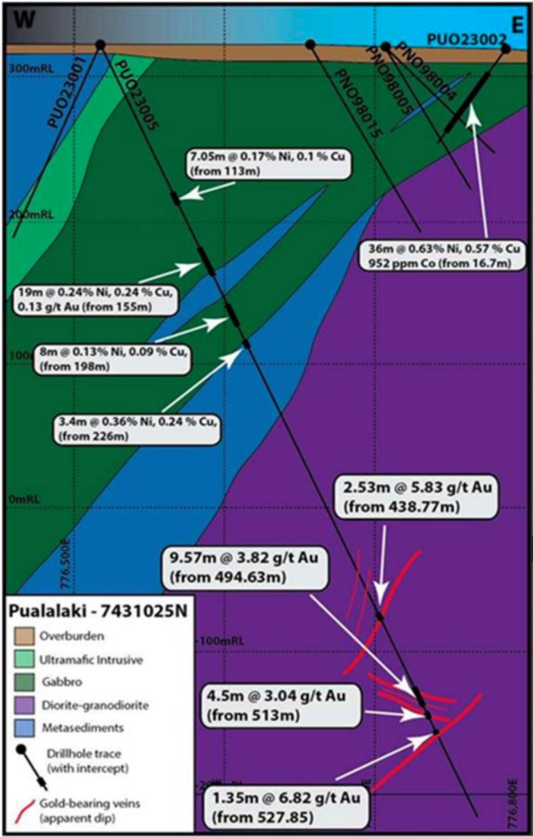
Puolalaki cross-section showing mineralised intercepts from PUO23005
